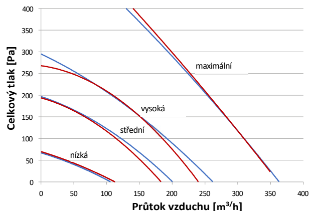
HRU-MinistAIR-325-H — Příklad do míst. — Výfuk
